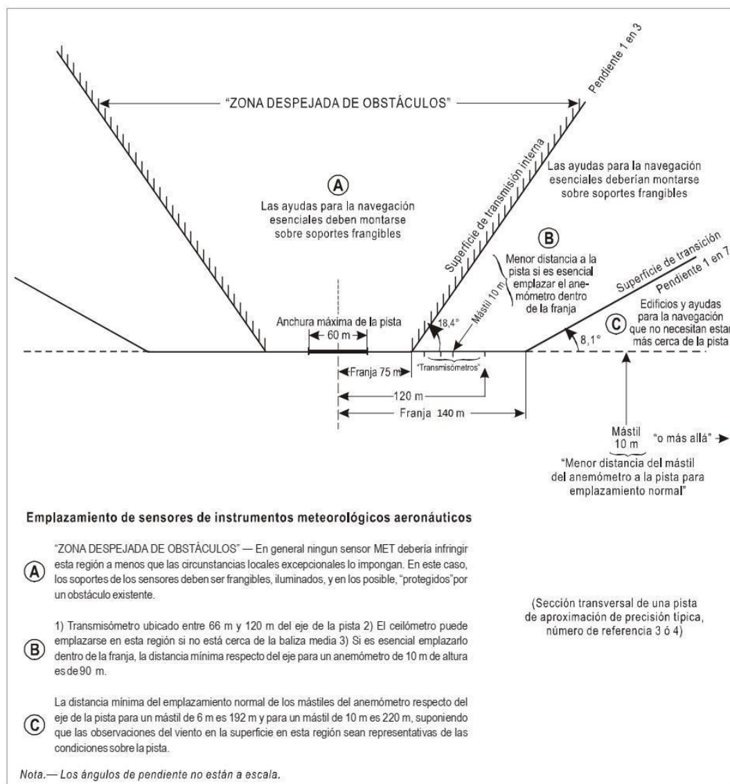
Figura E-1: Instalación de sensores para la observación meteorológica en el aeródromo.
